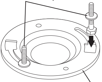
Boulons de 5/16 po de diamètre
